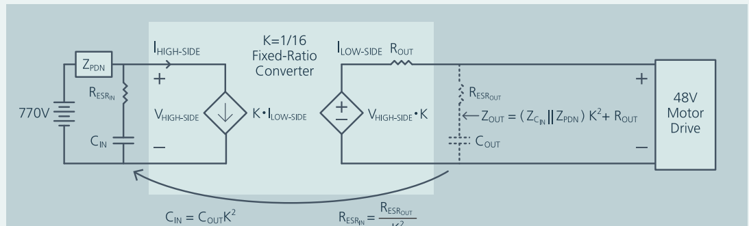
圖 6：阻抗反射可按 K^2 的因數降低有效電源的阻抗，從而可減少所需的電容。
